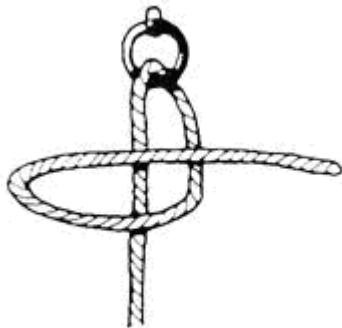
Stap 1 paardenknoop
